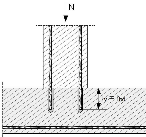
Bild 3: Endverankerung von Platten oder Balken
