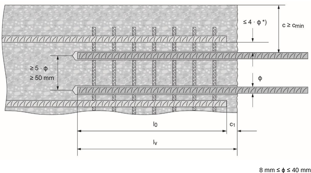
Bild 6: Abstände zwischen existierenden und nachträglich zu installierenden Bewehrungsstäben und Abstand zum (parallelen) Rand.
